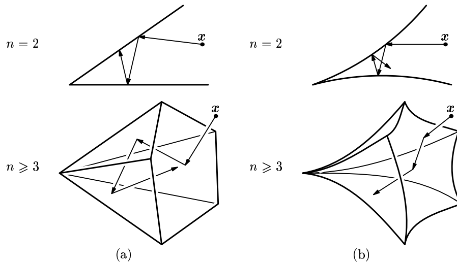
Рис. 6. «Малая» (a) и «большая» (b) задачи Синая
